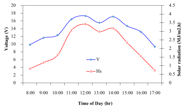
รูปที่ 3 ความสัมพันธ์ระหว่างพลังงานแสงอาทิตย์กับ แรงดันไฟฟ้าที่เครื่องผลิตได้(ข้อมูลการทดลองวันที่ 10)
