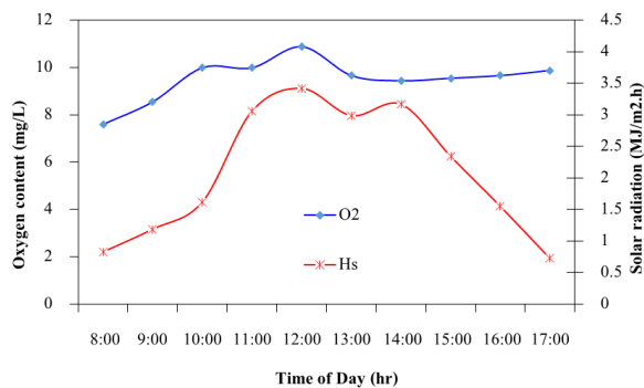
รูปที่ 2 ความสัมพันธ์ระหว่างพลังงานแสงอาทิตย์กับ ปริมาณออกซิเจนในน้ำ (ข้อมูลการทดลองวันที่ 10)
