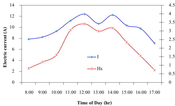
รูปที่ 4 ความสัมพันธ์ระหว่างพลังงานแสงอาทิตย์กับกระแสไฟฟ้าที่เครื่องผลิตไอดี (ข้อมูลการทดลองวันที่ 10)
