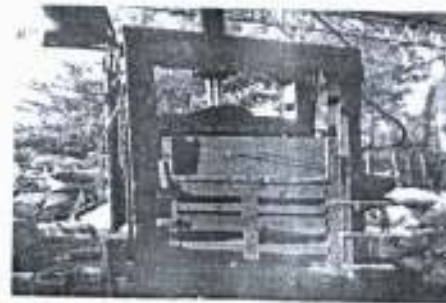
ภาพที่ 4 เครื่องอัดก้อนเหล็ก พลาสติก และกระดาษรีไซเคิล
