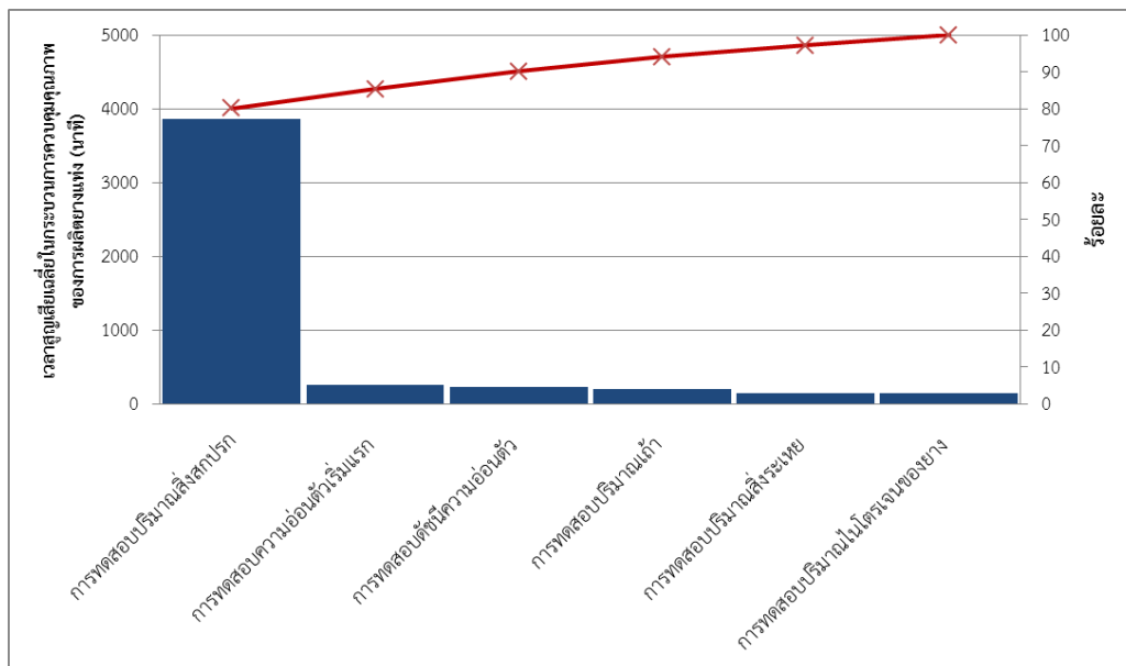
ภาพที่ 3 แผนภาพพารेटโตของเวลาสูญเสียเฉลี่ยในกระบวนการควบคุมคุณภาพของการผลิตยางแท่ง
