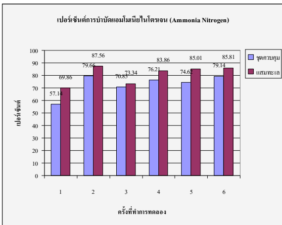
ภาพที่ 2 เปรียบเทียบเปอร์เซ็นต์การกำจัดแอมโมเนียไนโตรเจนในชุดการทดลองต่างๆ ตามระยะเวลาที่ทำการทดลอง
