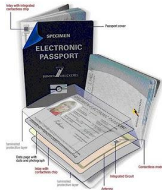
ภาพที่ 4 เทคโนโลยีอาร์เอฟไอดีในระบบหนังสือเดินทางอิเล็กทรอนิกส์
